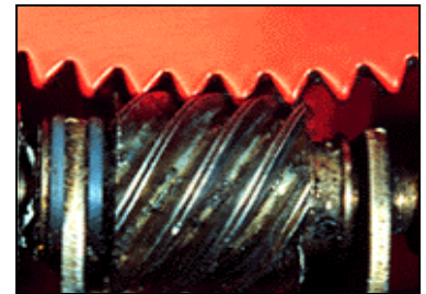
Engranajes sinfín
